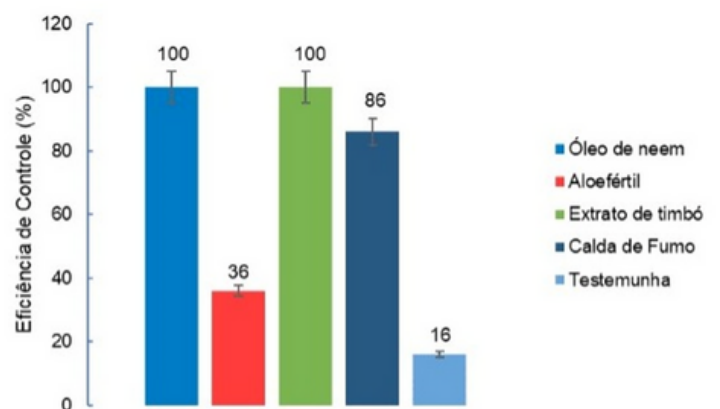
Figura 3. Eficiência de controle (%) de extratos botânicos no controle de lagartas de Tuta absoluta em plantas de tomateiro aos 10 dias após a aplicação. Barras com números seguidos pela mesma letra não diferem pelo teste de Tukey ( p < 0,05 ). Eficiência de controle calculada pela fórmula de Abbott (1925).
